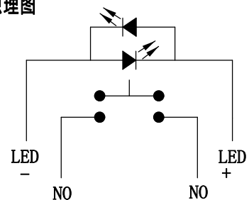
电气原理图
