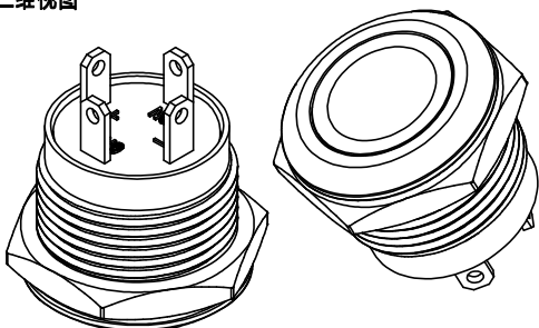
三维视图
