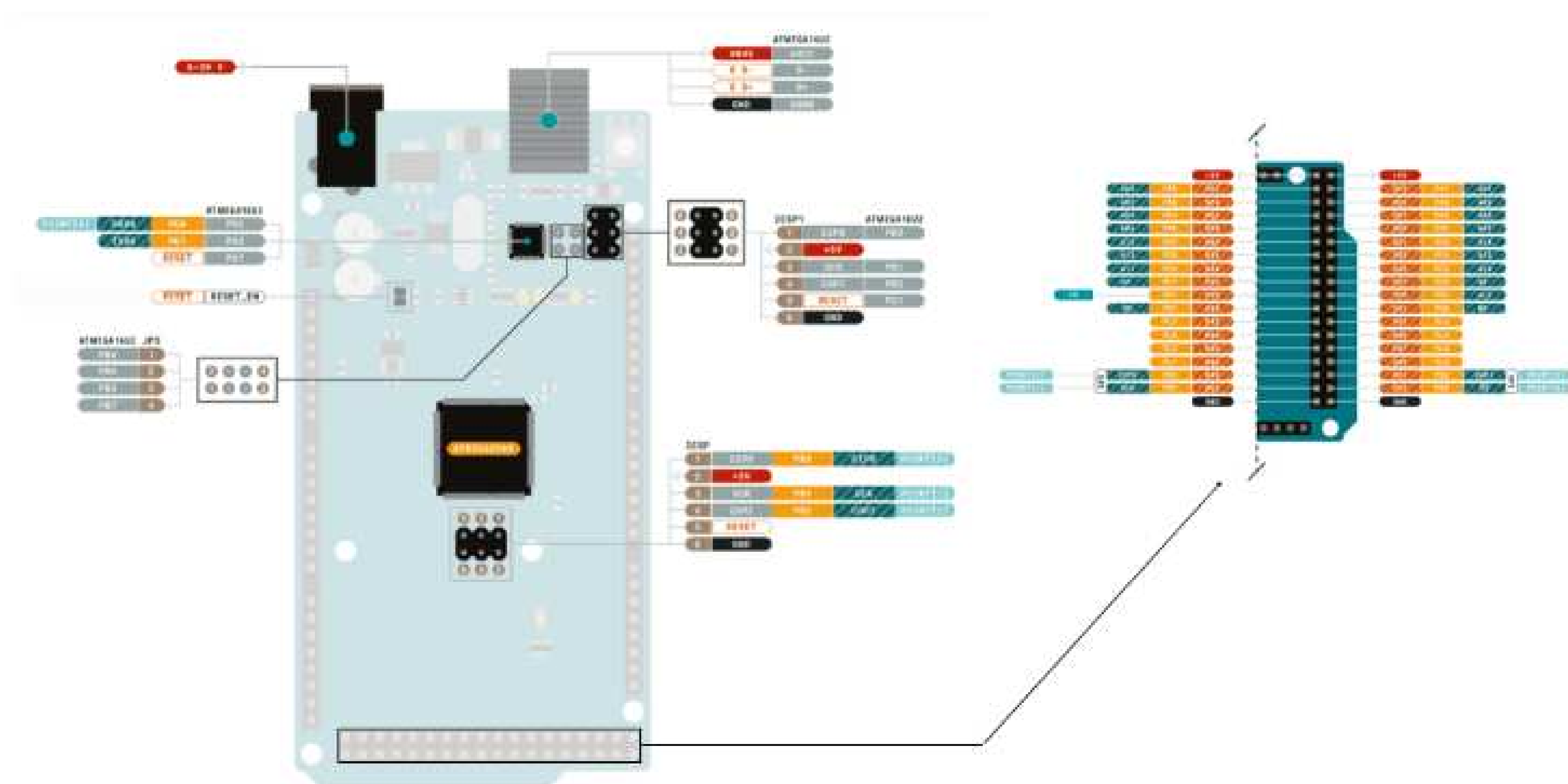
Arduino Mega 2560 Rev3 引脚布局
