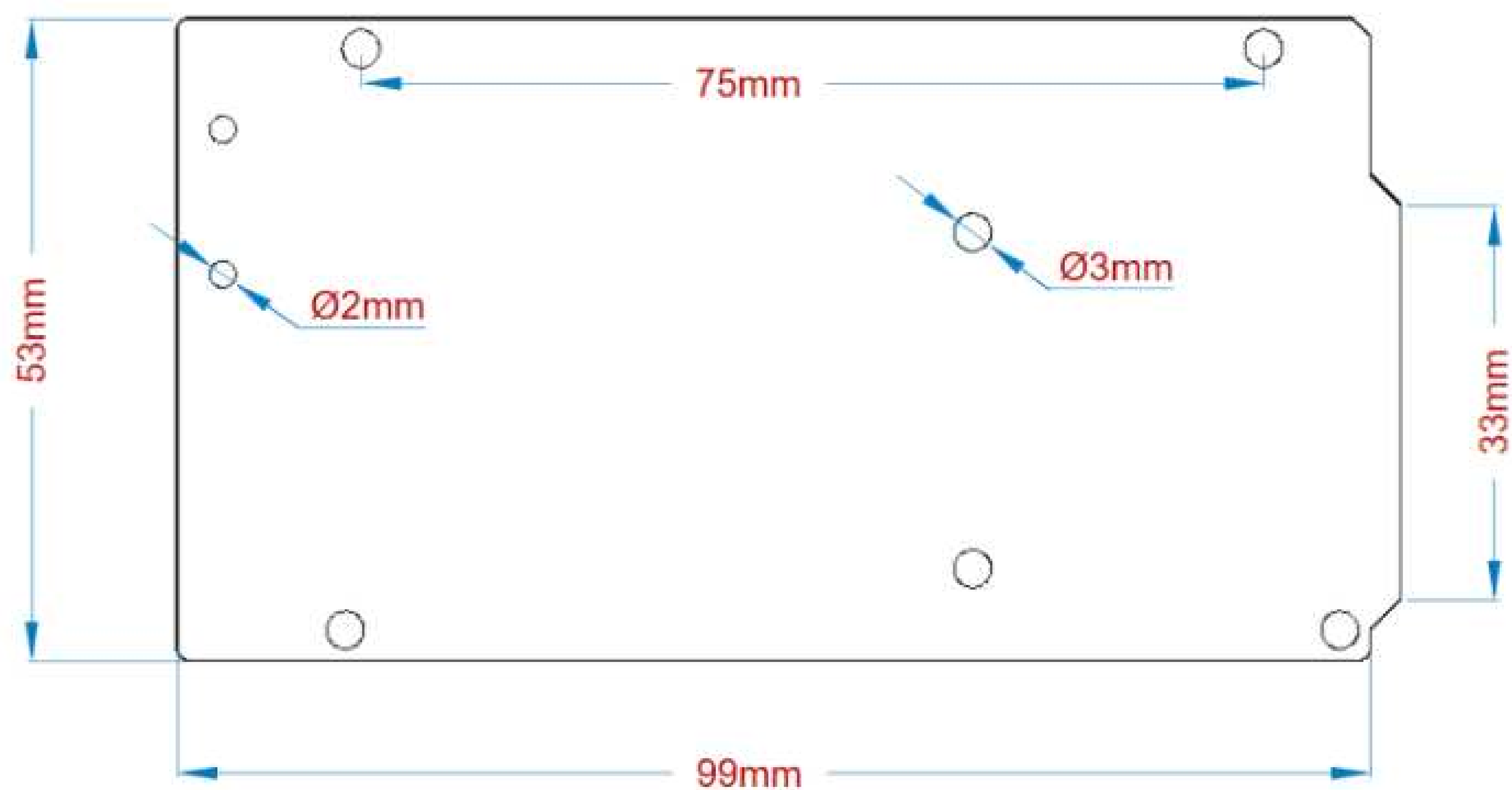
Arduino Mega 2560 Rev3 外形图
