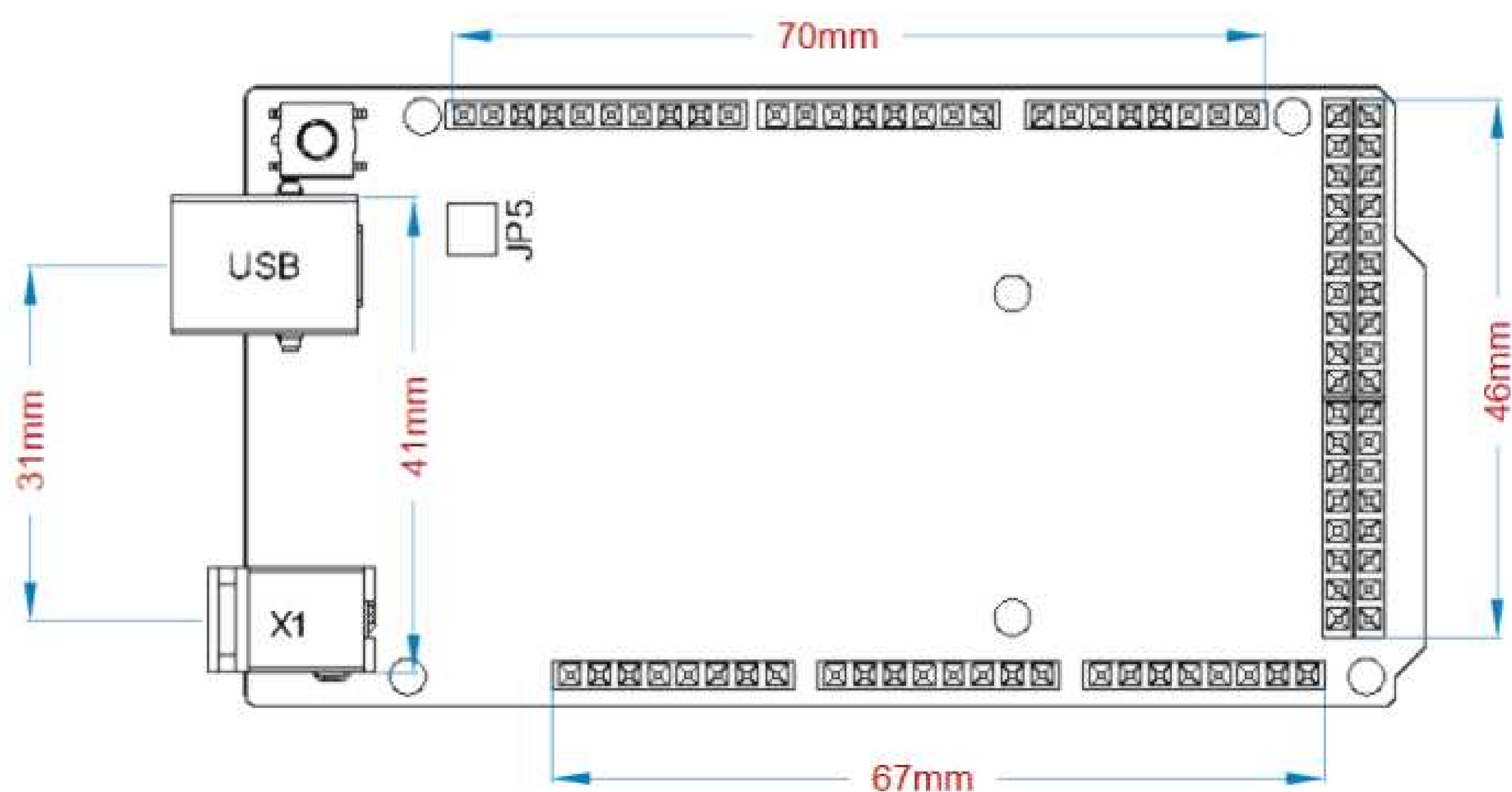
Arduino Mega 2560 Rev3 安装孔
