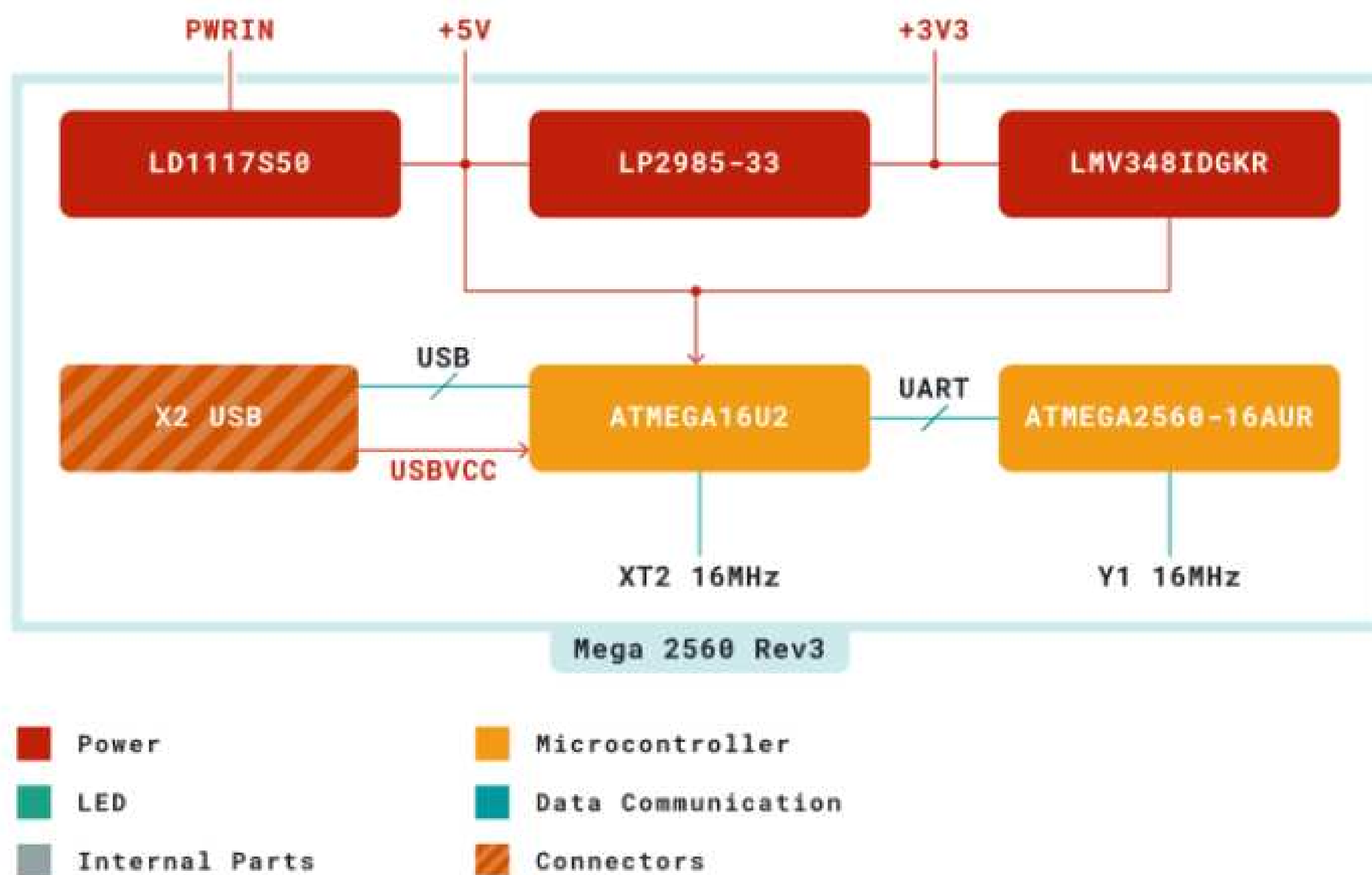
Arduino Mega 2560 Rev3 方框图
