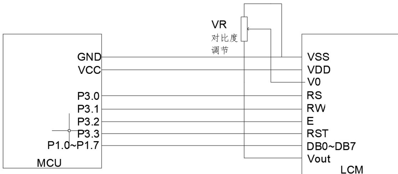
并行传输接线方法
