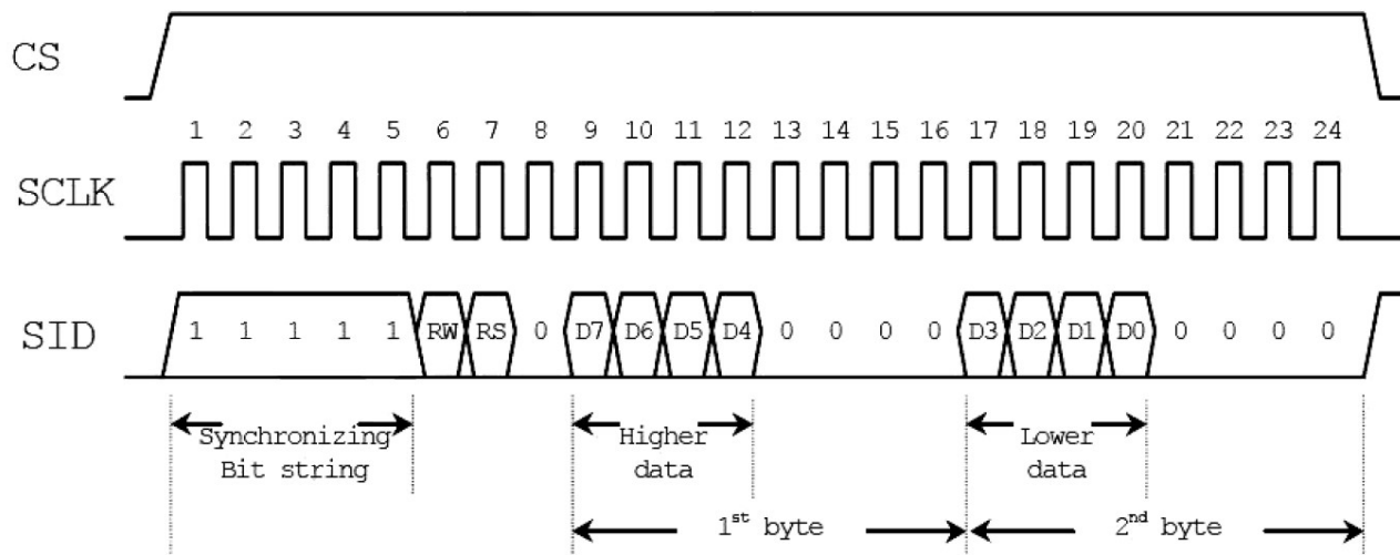
串行模式数据传输时序图
